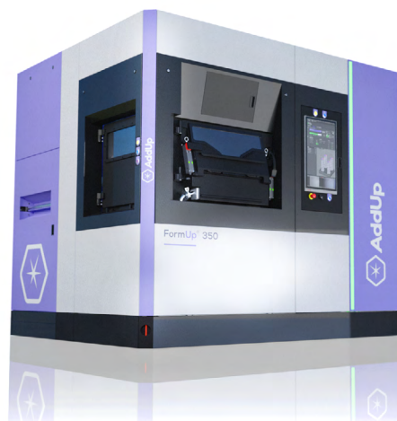
Fruit de deux ans de recherche avancée et de test dans les ateliers d'AddUp, FormUp 350 nouvelle génération est la solution permettant de relever les défis des industriels : sécurité, productivité, qualité et obsolescence. Crédit photo : AddUp
